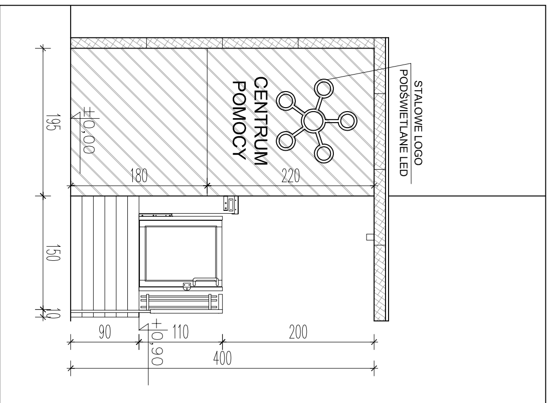
ELEWACJA ZACHODNIA
